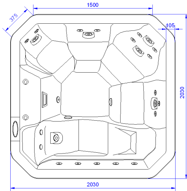
Σχέδιο A1: Κάτοψη
